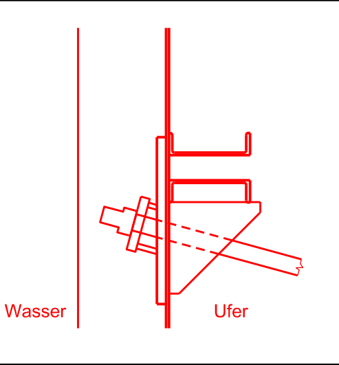
Prinzipskizze Ankeranschluss M ca. 1:10
