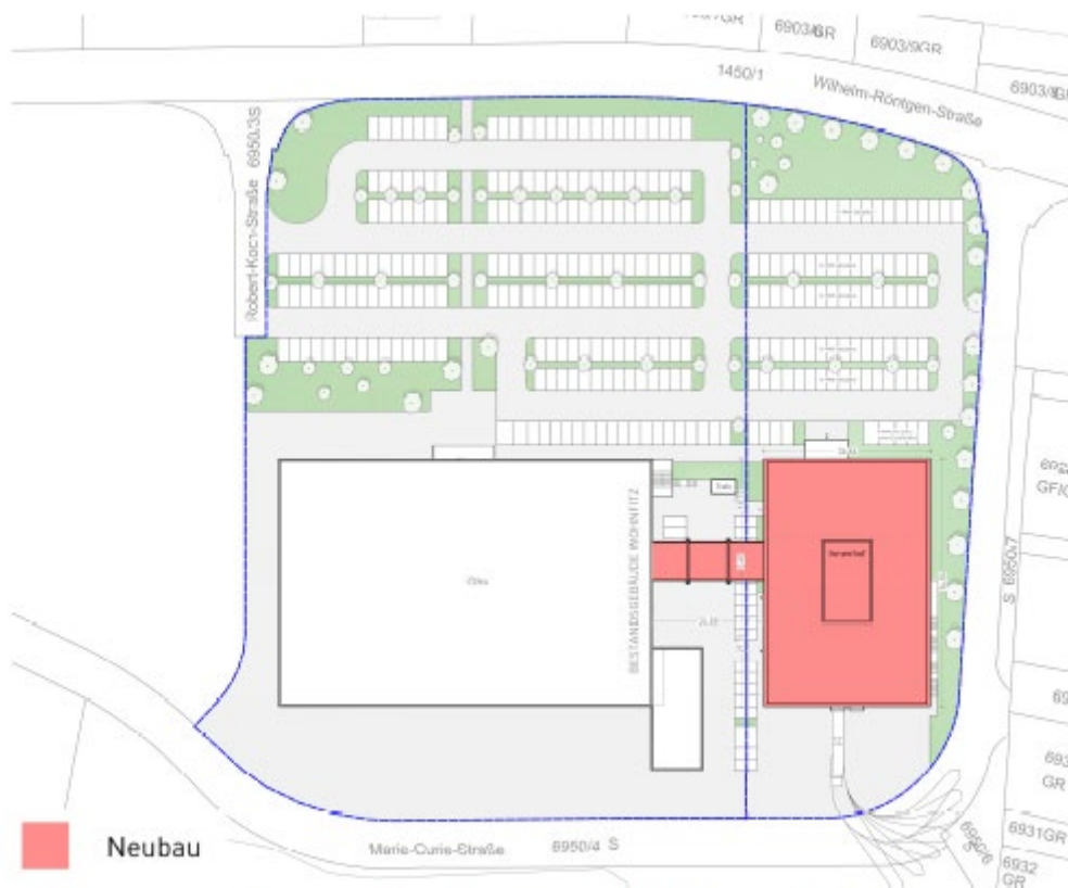
Abb. 2: Vorentwurf Erweiterung Möbelhaus Wohnfitz (Quelle: Fa. wohndfitz GmbH)
