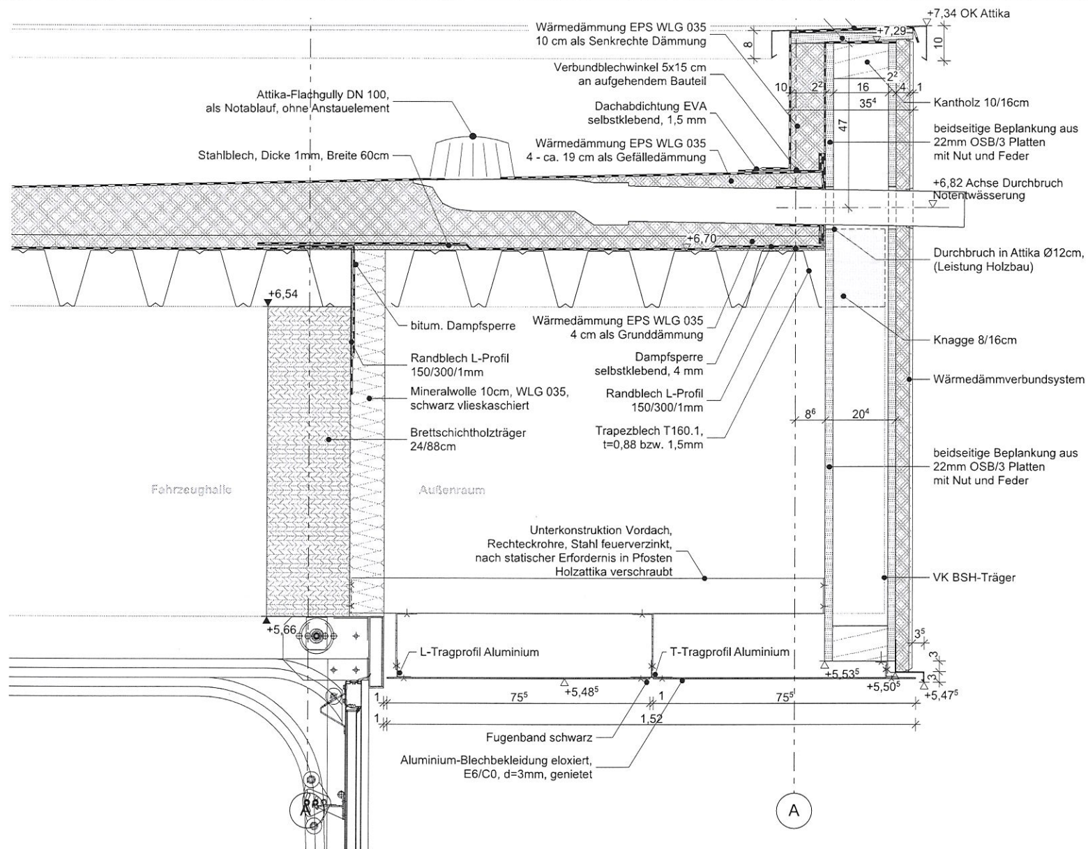
Detail Ausführung mit Untersichtverkleidung
